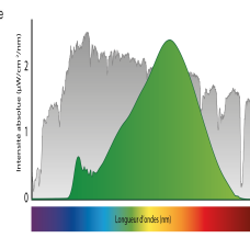
Spectre de lumière proche de la nature Pure-Z-NEO-LED Graphie gris : Spectre de la lumière du jour Graphie vert : Spectre typique ampoule Pure-Z-Retro-LED
