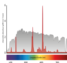
Spectre Typique d'une ampoule à économie d'énergie (fluo-compacte) Graphie gris : Spectre de la lumière du jour Graph rouge : Spectre typique ampoule fluo-compacte
