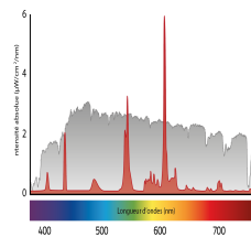
Grphe gris : Spectre de la lumière du jour Grphe rouge : Spectre typique ampoule fluo-compacte
