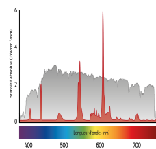
Graphes gris : Spectre de la lumière du jour Graph rouge : Spectre typique ampoule fluo-compacte
