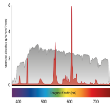
Spectre Typique d'une ampoule à économie d'énergie (fluo-compacte) Graphe gris : Spectre de la lumière du jour Graph rouge : Spectre typique ampoule fluo-compacte
